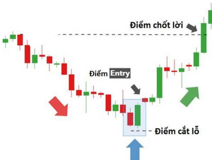
Mô hình nhấn chìm tăng xuất hiện ở cuối xu hướng Downtrend
